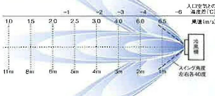
■冷風分布図
